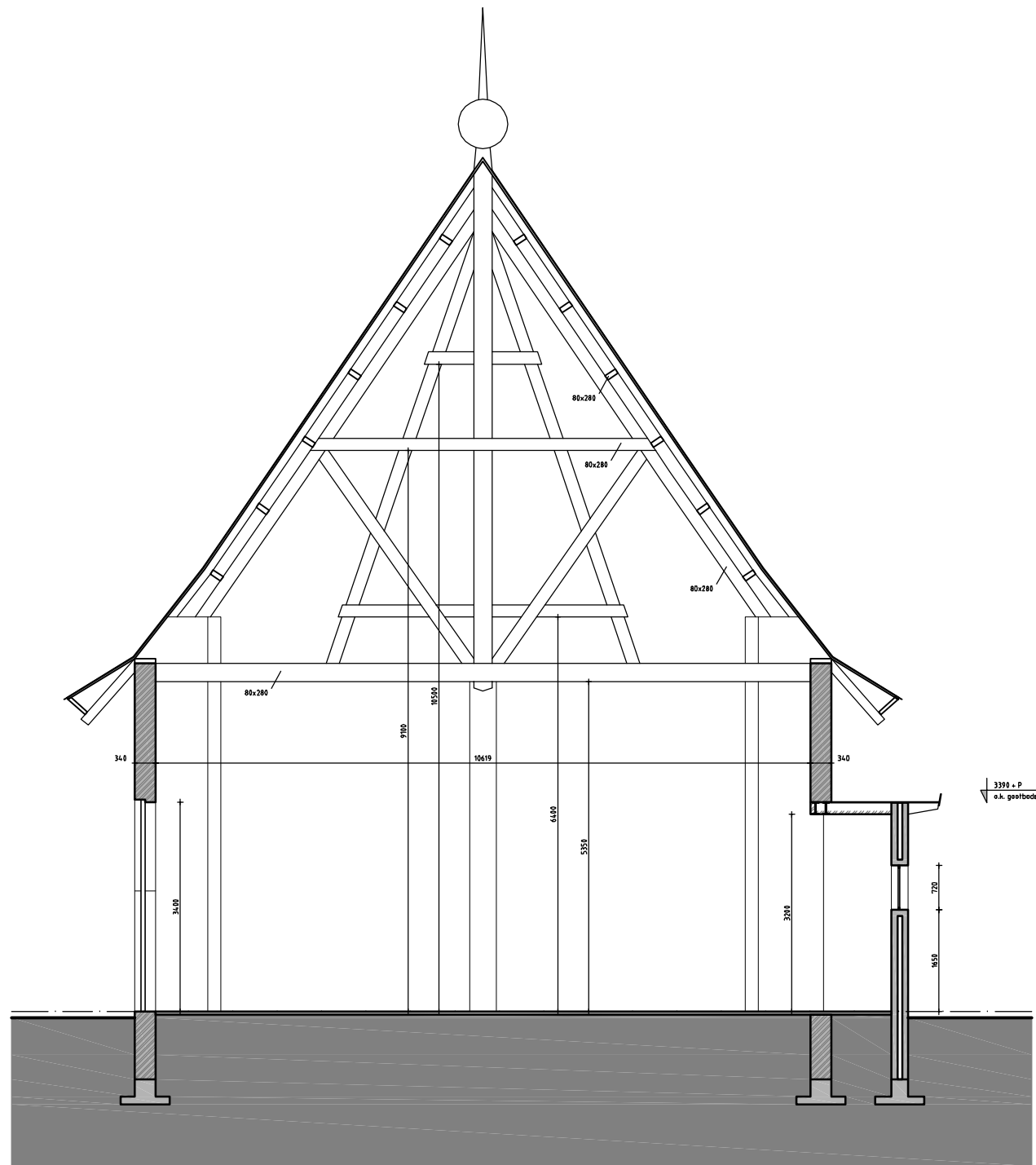
DOORSNEDE A-A
