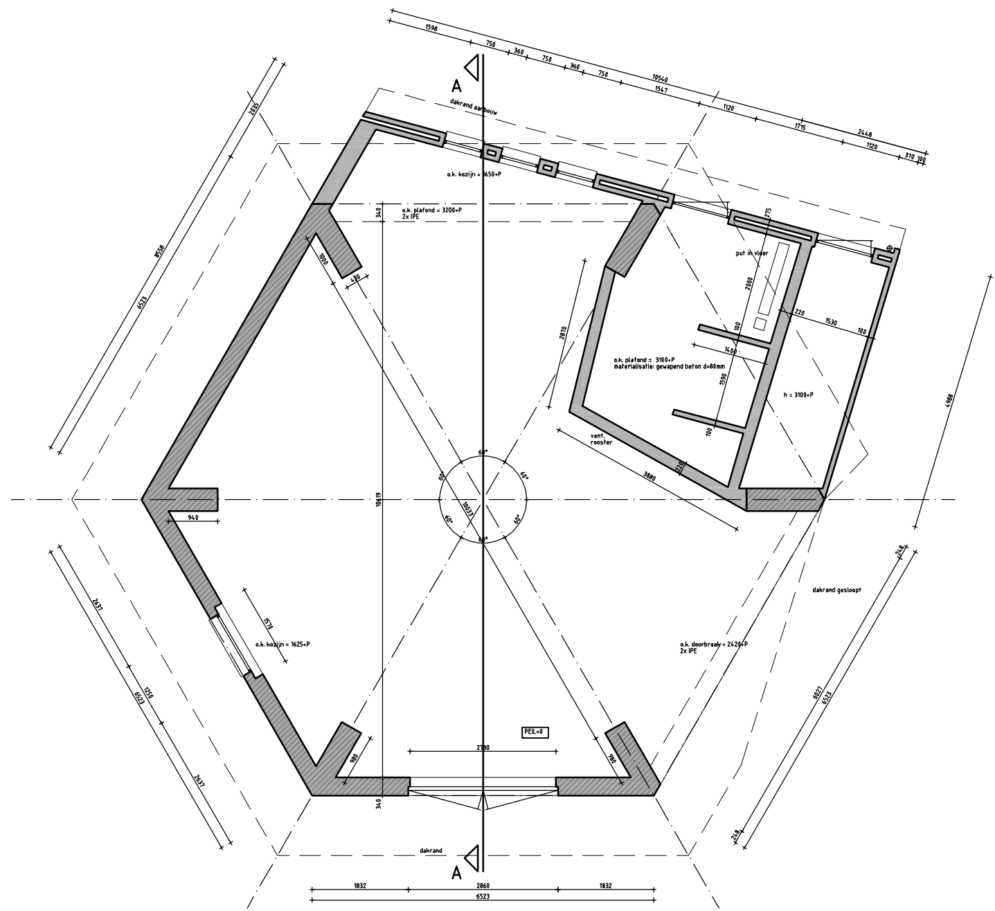
PLATTEGROND
